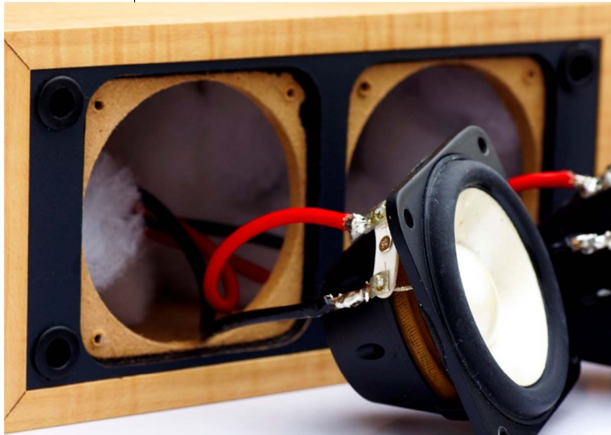
2.5 吋陶瓷披覆多重纖維紙盆全音域單體(PCC)
